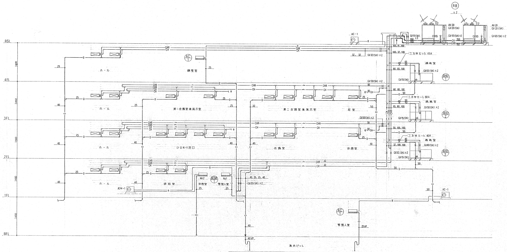
配管系統図
